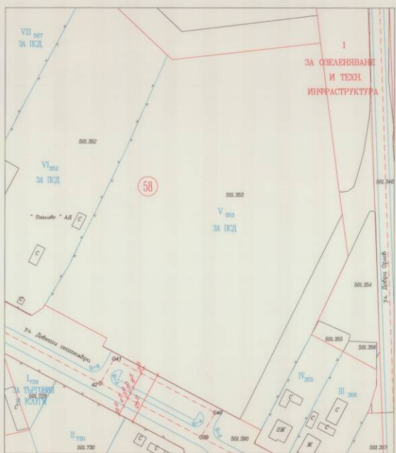
ПУП - ПЛАН ЗА РЕГУЛАЦИЯ НА УПИ V-353, КВ. 58, С. КРУШАРИ, ОБЩ. КРУШАРИ
