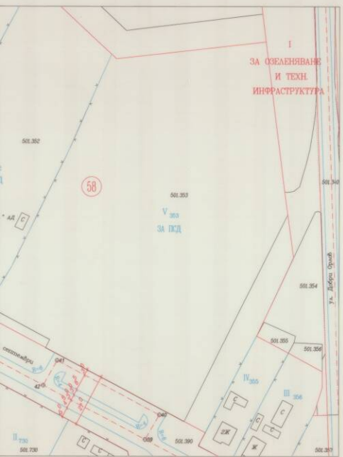
ИЗВАДКА ОТ КК И ОТ ДЕЙСТВИЯ ПУП - ПЛАН ЗА РЕГУЛАЦИЯ НА УПИ V-353, КВ. 58, С. КРУШАРИ, ОБЩ. КРУШАРИ
