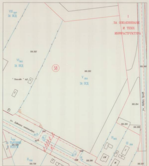
ИЗМЕНЕНИЕ НА ПУП - ПЛАН ЗА РЕГУЛАЦИЯ НА УПИ V-353, КВ. 58, С. КРУШАРИ, ОБЩ. КРУШАРИ
